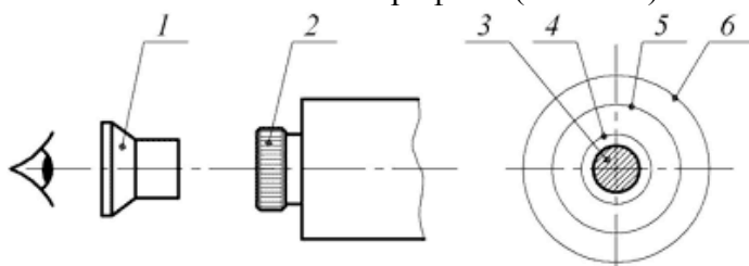
1 – вспомогательная лупа; 2 – окуляр коллиматора; 3 – входной зрачок объектива теодолита; 4 – оправа объектива теодолита; 5 – выходной зрачок объектива коллиматора; 6 – общее поле зрения окуляра коллиматора
